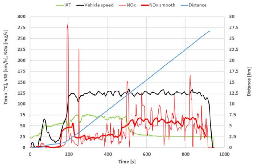
Figuur 4-30: Test bij een constante snelheid van 125 km/h met motorkalibratie 2 en koude start van 23-10-2018 op de testbaan. De inlaattemperatuur is tot t = 500 s rond 70\text{ }^{\circ}\text{C} . Daarna daalt de inlaattemperatuur naar 25\text{ }^{\circ}\text{C} en stijgt de \text{NO}_x emissie van ongeveer 25 naar 50-65 mg/s. Dit duidt op een daling van de hoeveelheid EGR.
